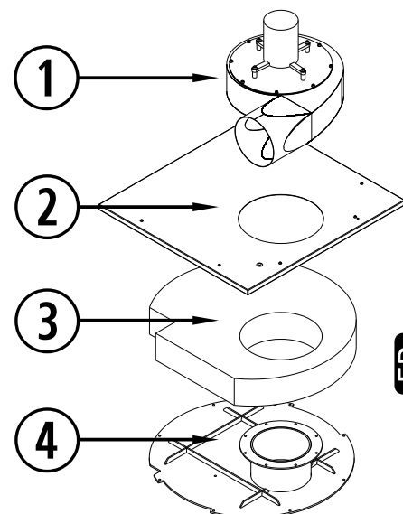
Schéma 18
