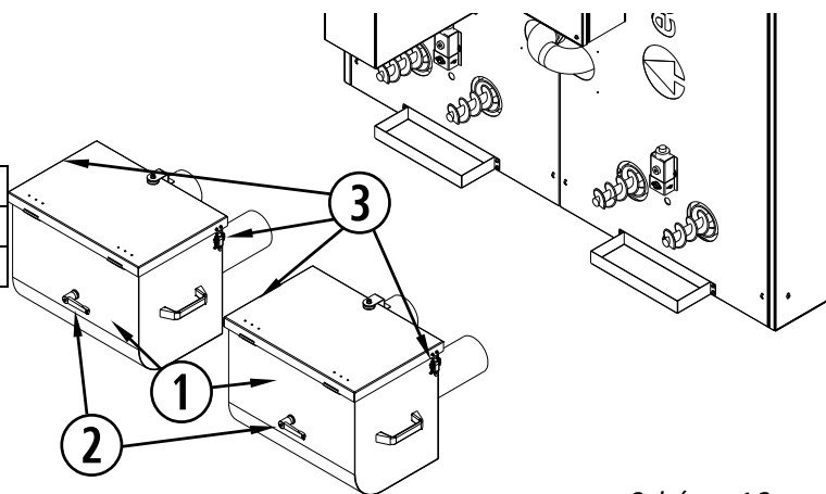
Schéma 16
