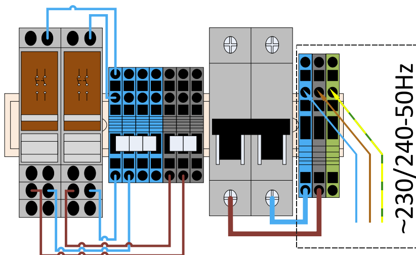
Schéma 7
