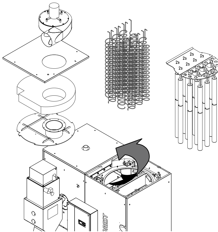
Schéma 17
