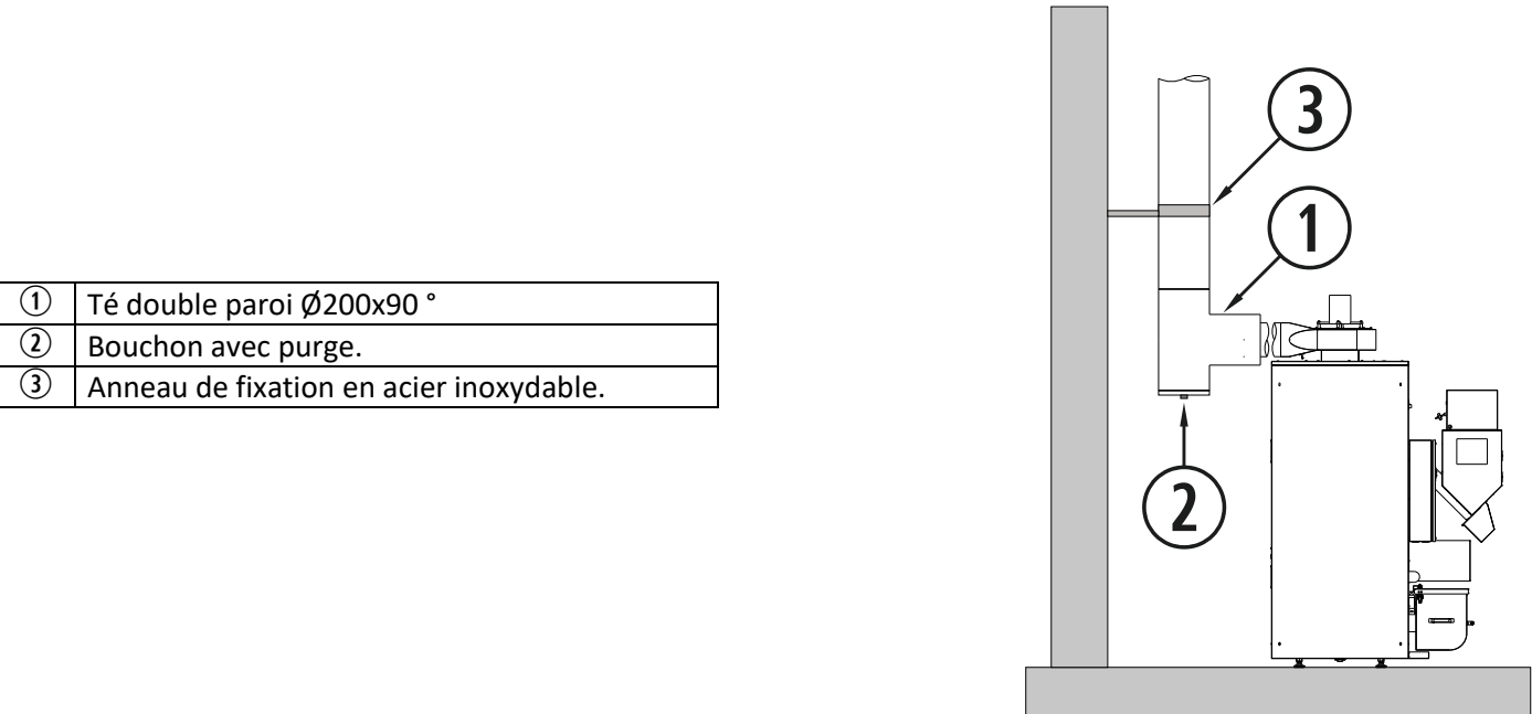
Schéma 10
