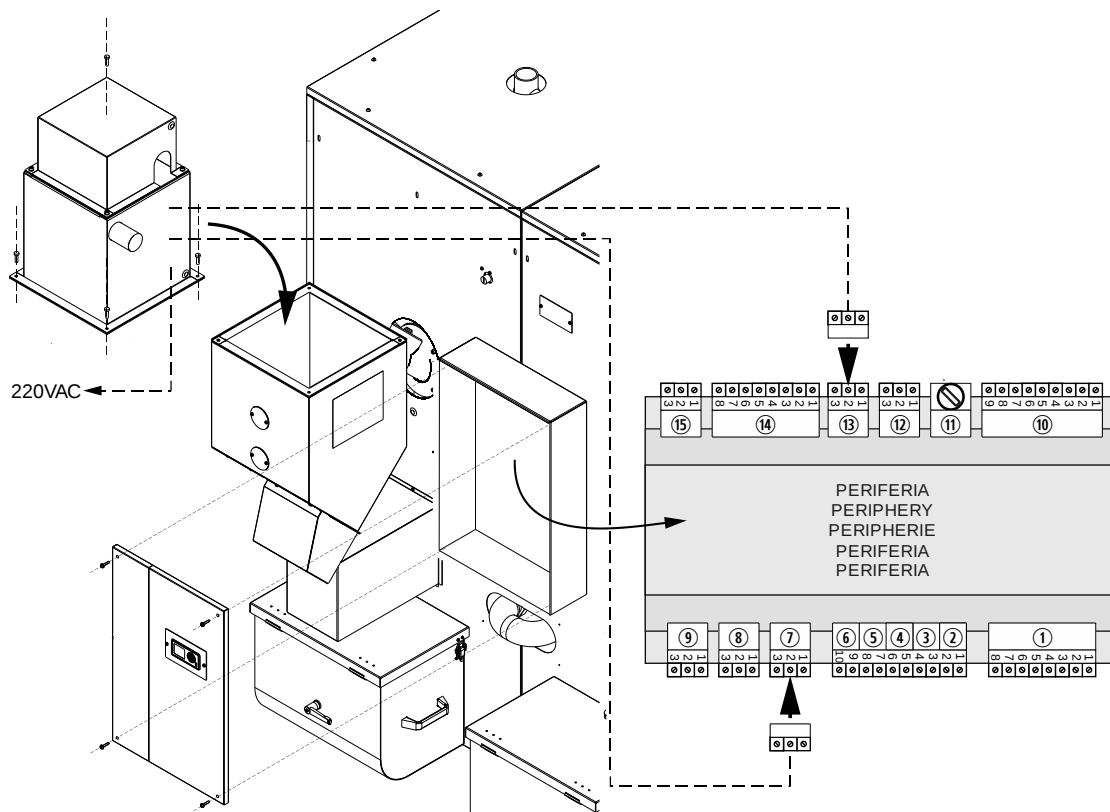
Schéma 3
